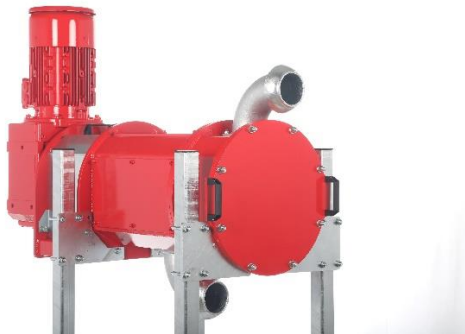
Bild 3: Innovative Separationstechnik: der Pressschneckenseparator XSplit.
